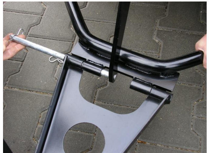
6. Čep radlice provlékněte i táhlem.
