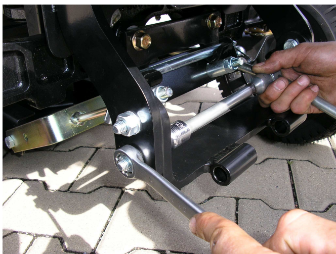
8. Nasad'te střední díl rámu a zajistěte šrouby a dotáhněte
