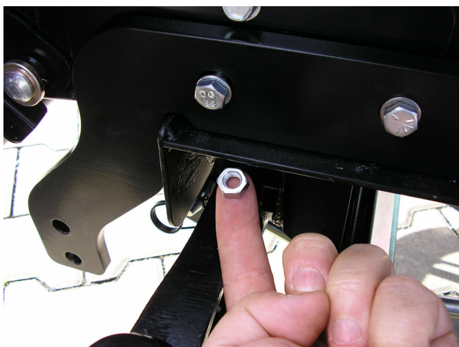
6. Postup opakujte i na levé straně traktoru zajistěte čepem a závlačkami.
